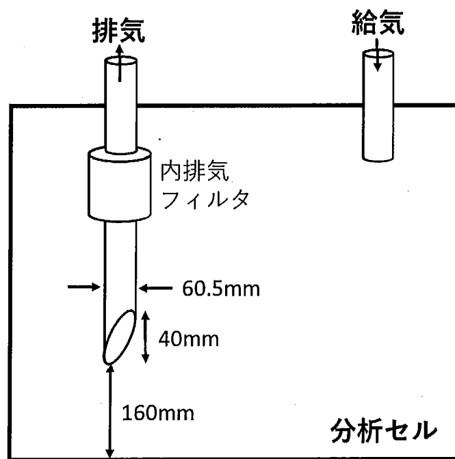
別図-1 分析セルの排気配管の構造
